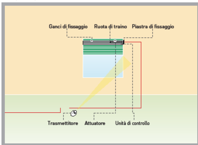
Esempio d'impianto LOOP50/35
